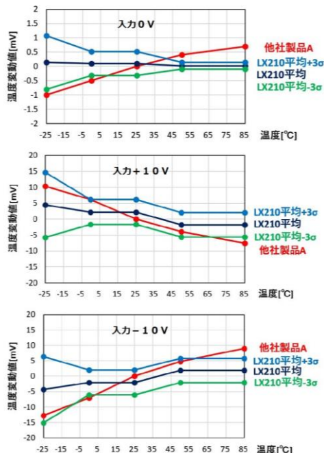
温度ドリフト (出力電圧) G=1、-25°C~85°C
