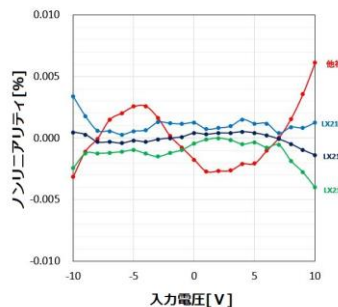
非直線性(ノンリニアリティ)[%] 3σデータ (回掃直線との差)/フルスケール(20V)×100
